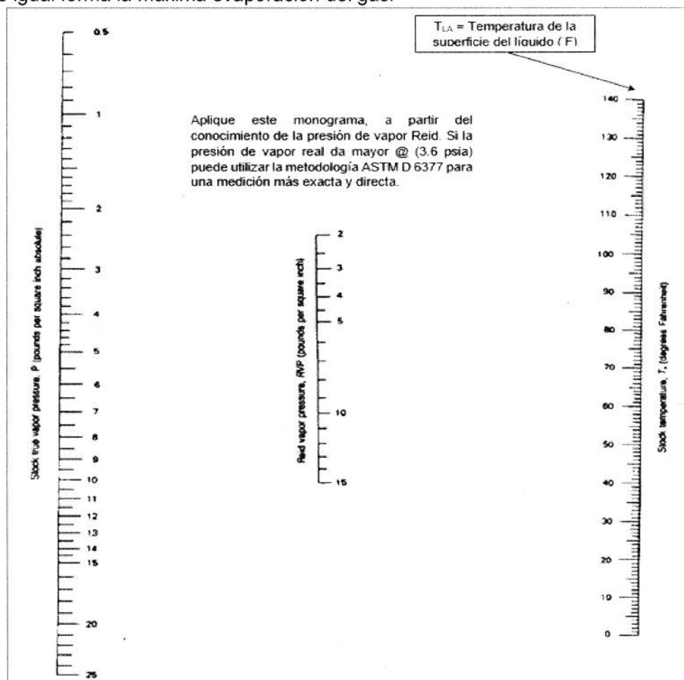
Figura. 7.1-13a Nomograma para cálculo de la presión de vapor real.
