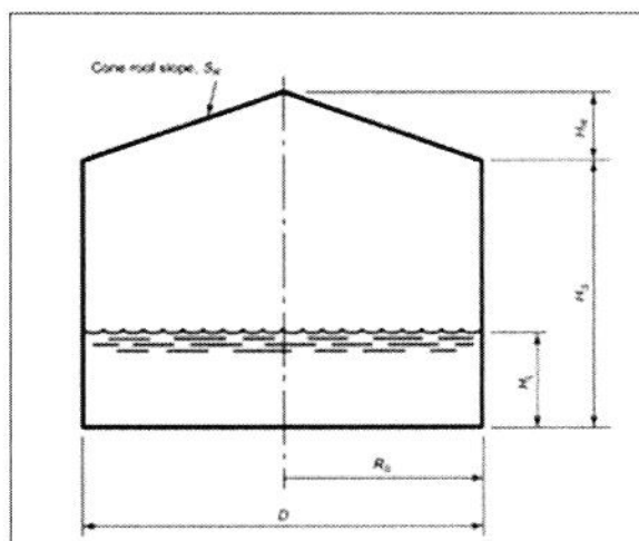
Dimensiones en un tanque de techo cónico.
